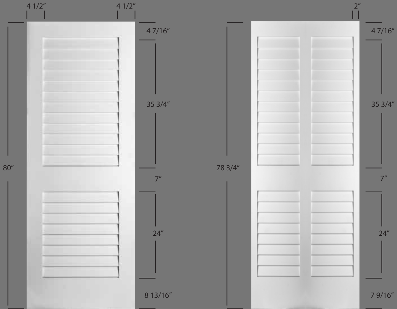
730 Door: Louver/Louver
